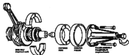
#832-209(6206)のベアリングを抜く場合
